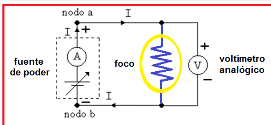
Figura 1.2. Dispositivo experimental.
