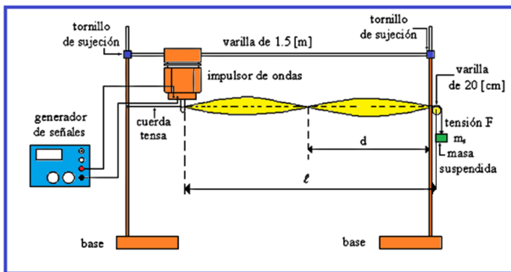
Figura 7.1. Dispositivo experimental.
