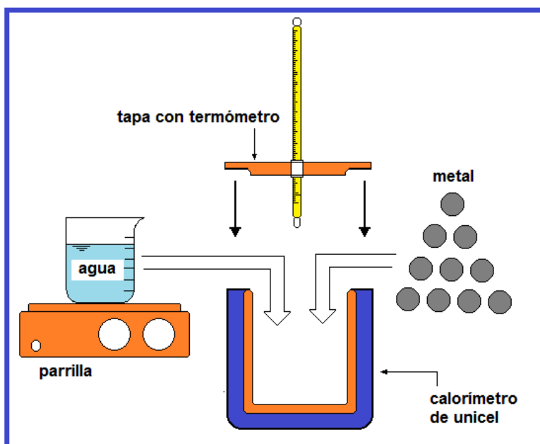
Figura 6.1. Dispositivo experimental.
