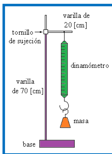
Figura 2.1. Dispositivo experimental del dinamómetro.
