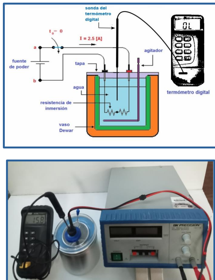
Figura 5.1. Dispositivo experimental.
