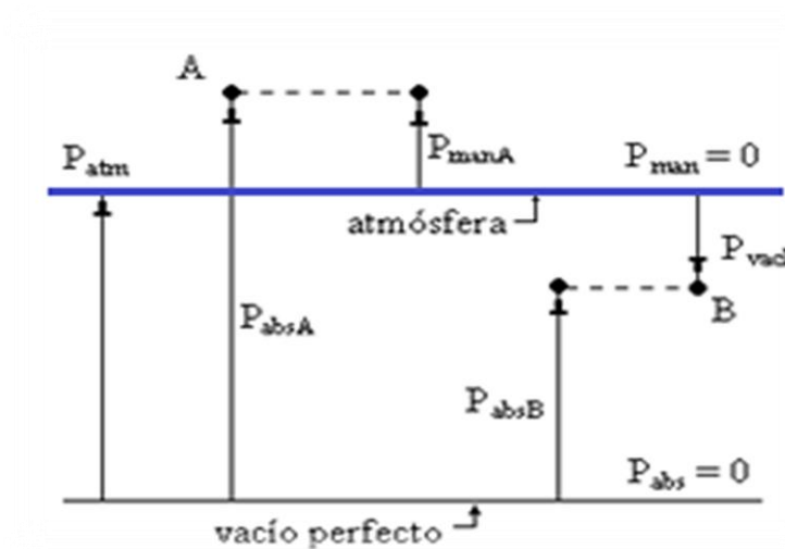
Figura 4.2. Presión manométrica, presión vacuométrica y presión absoluta.
