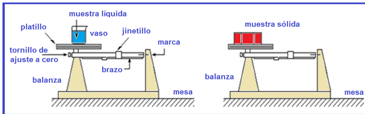
Figura 3.1. Diagrama de medición de muestras sólidas y líquidas.
